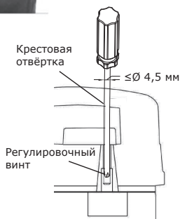
Рис. 3 Регулировочный винт колодезной насосной установки AQUATRON
