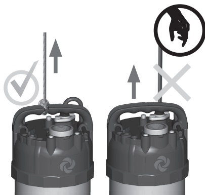
Рис. 2 Подъём насоса
