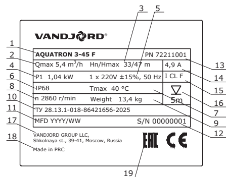
Рис. 1 Фирменная табличка
